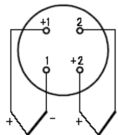
dvojitý termočlánek
